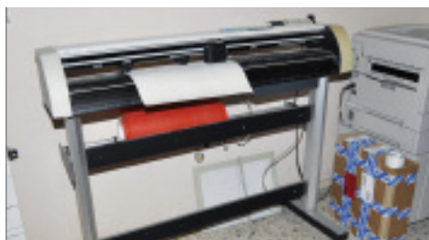
Die Schneidemaschine Mimaki überträgt Schrift auf eine Tiefstrahlfolie.
