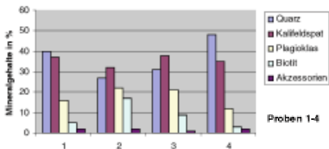
Mineralische Zusammensetzung des Kugelgranites Ruskiavouri
