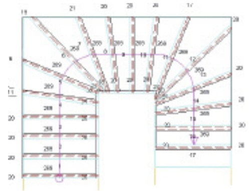
StonePro/CAD ermöglicht die schnelle Konstruktion von Treppen.
