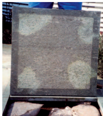
Bleibende farbliche Veränderungen in einem Naturwerksteinbelag aus ANDEER, verlegt auf Mörtelbatzen.
