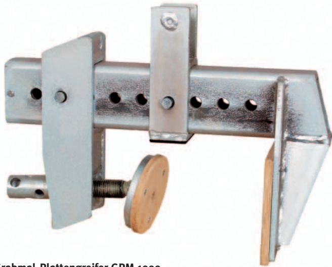
Grabmal-Plattengreifer GPM 1000.
